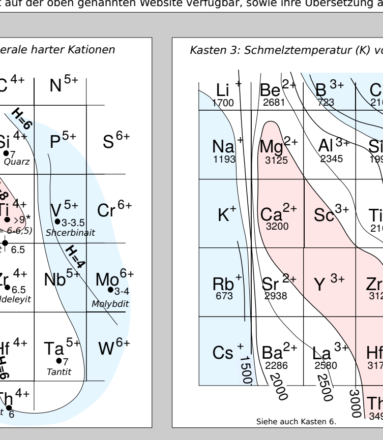
Eine Periodentabelle der Elemente und ihrer Ionen für Geowissenschaftler Version 4.8e © 2012 L. Bruce Railsback, Department of Geology, University of Georgia, Athens, Georgia, 30602-2501 U.S.A (rlsbk@gly.uga.edu). Übersetzung von: Stephan Lenk, Institut für Geologie, TU Bergakademie Freiberg (stephan-lenk@student.tu-freiberg.de) 2014. Siehe http://www.gly.uga.edu/railsback/PT.html für Aktualisierungen und mehr Informationen. Version 4.6 dieser Tabelle wurde als Abbildung 1 des folgenden Artikels veröffentlicht: Railsback, L.B., 2003, An Earth Scientist's Periodic Table of the Elements and Their Ions: Geology v. 31, no. 9, p. 737-740. Die Veröffentlichung der Version 4.6 in Geology wurde von der National Science Foundation Grant DUE 02-03115 unterstützt. Version 4.7 wurde 2004 in der Geological Society of America's Map and Chart Series als Objekt MCH092 veröffentlicht. Version 4.8 ist auf der oben genannten Website verfügbar, sowie ihre Übersetzung auf Spanisch, Chinesisch und Deutsch.
