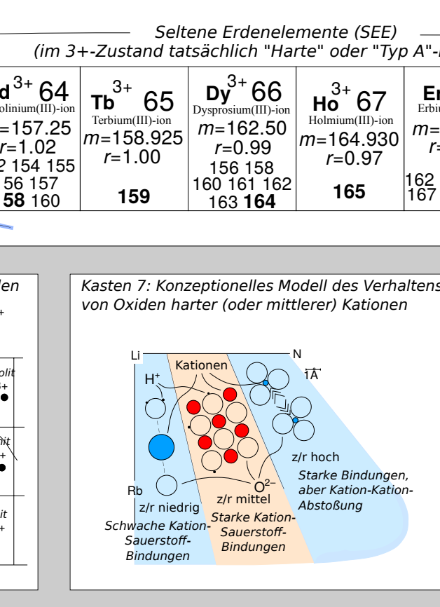
Eine Periodentabelle der Elemente und ihrer Ionen für Geowissenschaftler Version 4.8e © 2012 L. Bruce Railsback, Department of Geology, University of Georgia, Athens, Georgia, 30602-2501 U.S.A (rlsbk@gly.uga.edu). Übersetzung von: Stephan Lenk, Institut für Geologie, TU Bergakademie Freiberg (stephan-lenk@student.tu-freiberg.de) 2014. Siehe http://www.gly.uga.edu/railsback/PT.html für Aktualisierungen und mehr Informationen. Version 4.6 dieser Tabelle wurde als Abbildung 1 des folgenden Artikels veröffentlicht: Railsback, L.B., 2003, An Earth Scientist's Periodic Table of the Elements and Their Ions: Geology v. 31, no. 9, p. 737-740. Die Veröffentlichung der Version 4.6 in Geology wurde von der National Science Foundation Grant DUE 02-03115 unterstützt. Version 4.7 wurde 2004 in der Geological Society of America's Map and Chart Series als Objekt MCH092 veröffentlicht. Version 4.8 ist auf der oben genannten Website verfügbar, sowie ihre Übersetzung auf Spanisch, Chinesisch und Deutsch.
