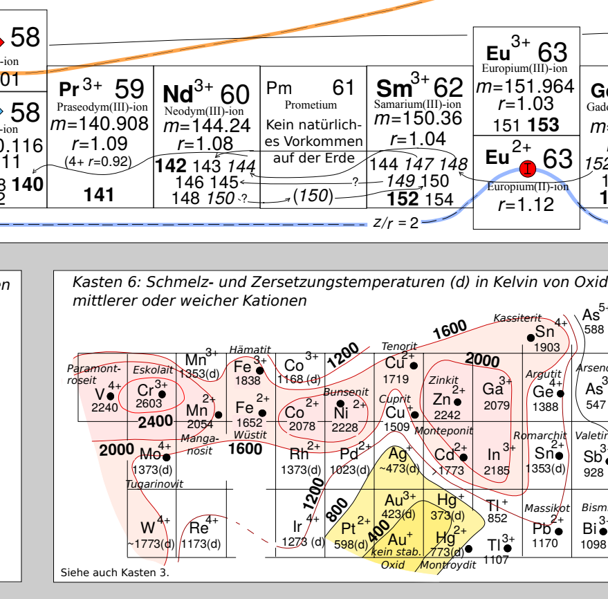
Eine Periodentabelle der Elemente und ihrer Ionen für Geowissenschaftler Version 4.8e © 2012 L. Bruce Railsback, Department of Geology, University of Georgia, Athens, Georgia, 30602-2501 U.S.A (rlsbk@gly.uga.edu). Übersetzung von: Stephan Lenk, Institut für Geologie, TU Bergakademie Freiberg (stephan-lenk@student.tu-freiberg.de) 2014. Siehe http://www.gly.uga.edu/railsback/PT.html für Aktualisierungen und mehr Informationen. Version 4.6 dieser Tabelle wurde als Abbildung 1 des folgenden Artikels veröffentlicht: Railsback, L.B., 2003, An Earth Scientist's Periodic Table of the Elements and Their Ions: Geology v. 31, no. 9, p. 737-740. Die Veröffentlichung der Version 4.6 in Geology wurde von der National Science Foundation Grant DUE 02-03115 unterstützt. Version 4.7 wurde 2004 in der Geological Society of America's Map and Chart Series als Objekt MCH092 veröffentlicht. Version 4.8 ist auf der oben genannten Website verfügbar, sowie ihre Übersetzung auf Spanisch, Chinesisch und Deutsch.
