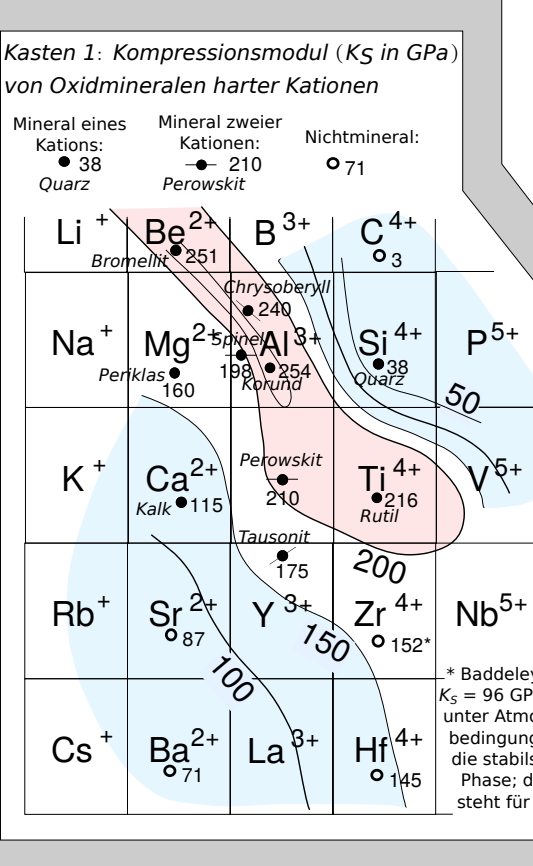
Eine Periodentabelle der Elemente und ihrer Ionen für Geowissenschaftler Version 4.8e © 2012 L. Bruce Railsback, Department of Geology, University of Georgia, Athens, Georgia, 30602-2501 U.S.A (rlsbk@gly.uga.edu). Übersetzung von: Stephan Lenk, Institut für Geologie, TU Bergakademie Freiberg (stephan-lenk@student.tu-freiberg.de) 2014. Siehe http://www.gly.uga.edu/railsback/PT.html für Aktualisierungen und mehr Informationen. Version 4.6 dieser Tabelle wurde als Abbildung 1 des folgenden Artikels veröffentlicht: Railsback, L.B., 2003, An Earth Scientist's Periodic Table of the Elements and Their Ions: Geology v. 31, no. 9, p. 737-740. Die Veröffentlichung der Version 4.6 in Geology wurde von der National Science Foundation Grant DUE 02-03115 unterstützt. Version 4.7 wurde 2004 in der Geological Society of America's Map and Chart Series als Objekt MCH092 veröffentlicht. Version 4.8 ist auf der oben genannten Website verfügbar, sowie ihre Übersetzung auf Spanisch, Chinesisch und Deutsch.
