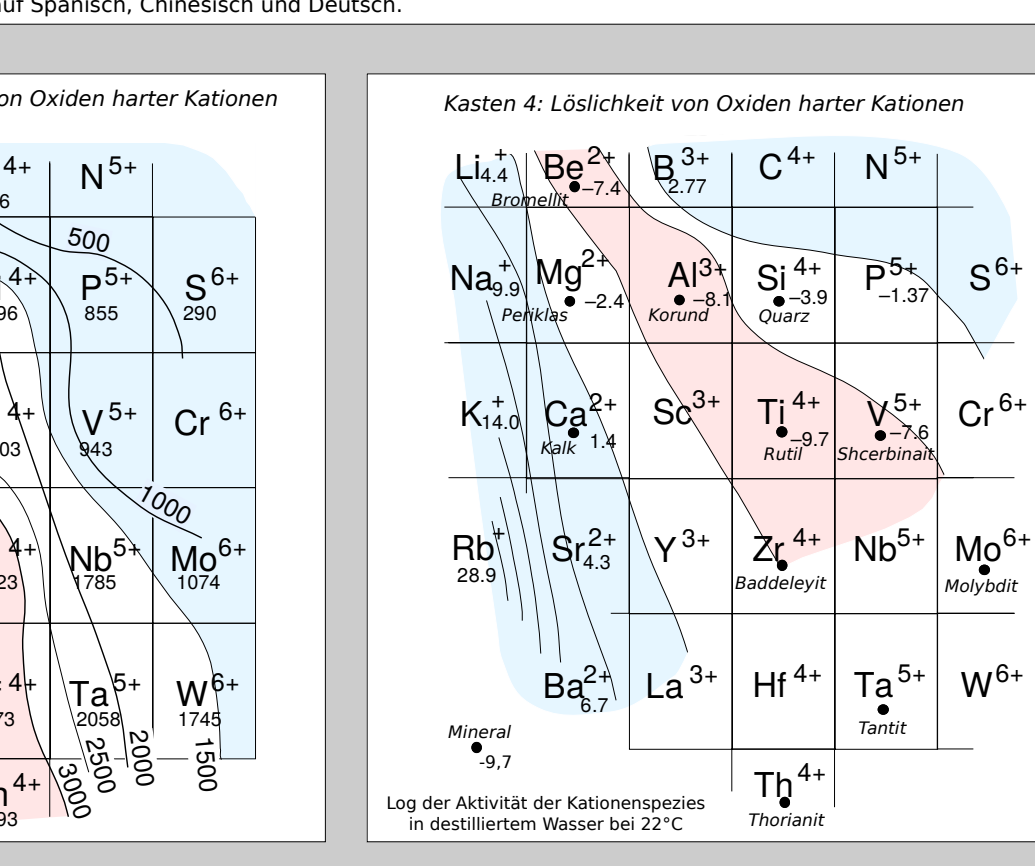
Eine Periodentabelle der Elemente und ihrer Ionen für Geowissenschaftler Version 4.8e © 2012 L. Bruce Railsback, Department of Geology, University of Georgia, Athens, Georgia, 30602-2501 U.S.A (rlsbk@gly.uga.edu). Übersetzung von: Stephan Lenk, Institut für Geologie, TU Bergakademie Freiberg (stephan-lenk@student.tu-freiberg.de) 2014. Siehe http://www.gly.uga.edu/railsback/PT.html für Aktualisierungen und mehr Informationen. Version 4.6 dieser Tabelle wurde als Abbildung 1 des folgenden Artikels veröffentlicht: Railsback, L.B., 2003, An Earth Scientist's Periodic Table of the Elements and Their Ions: Geology v. 31, no. 9, p. 737-740. Die Veröffentlichung der Version 4.6 in Geology wurde von der National Science Foundation Grant DUE 02-03115 unterstützt. Version 4.7 wurde 2004 in der Geological Society of America's Map and Chart Series als Objekt MCH092 veröffentlicht. Version 4.8 ist auf der oben genannten Website verfügbar, sowie ihre Übersetzung auf Spanisch, Chinesisch und Deutsch.
